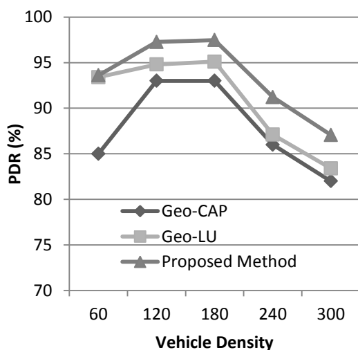
شکل (۵): نرخ تحویل بسته در Geo-CAP, Geo-LU و روش پیشنهادی با افزایش تعداد خودروها
