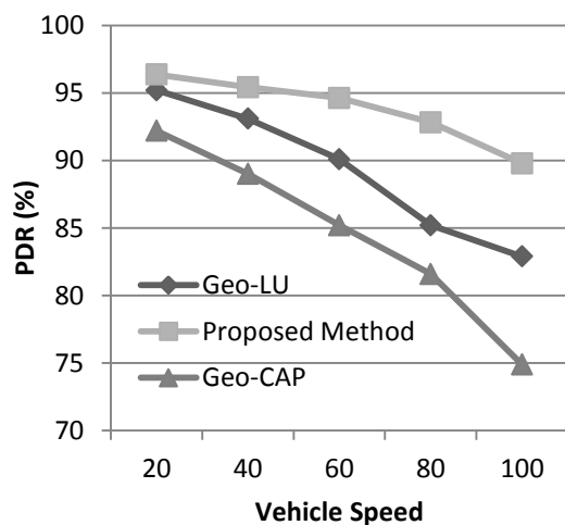
شکل (۷): نرخ تحویل بسته در روش پیشنهادی و الگوریتم‌های Geo-LU و Geo-CAP با افزایش سرعت گره‌ها
