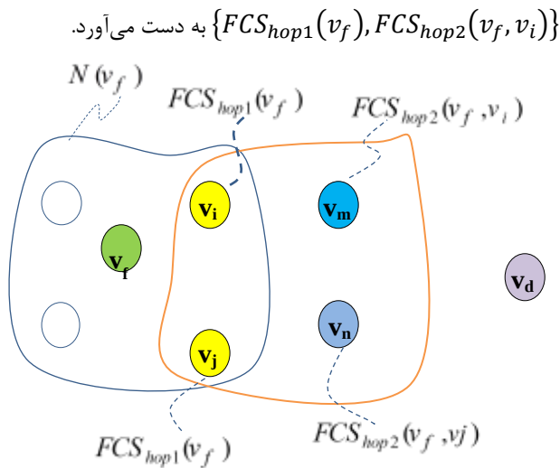
شکل (۱): کاندیدهای یک گامی و دو گامی گره v_f در الگوریتم Geo-LU
