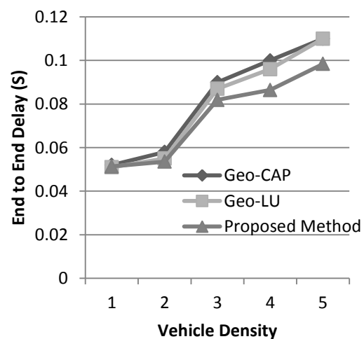
شکل (۸): تأخیر انتها به انتها در روش پیشنهادی، Geo-LU و Geo-CAP با افزایش تعداد خودروها
