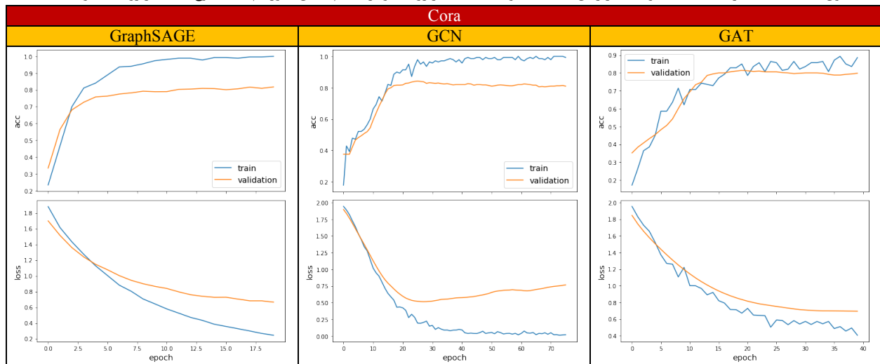
جدول (۷): مقایسه جاسازی گراف هنگام اعمال الگوریتم های متنوع GNN بر روی مجموعه داده Cora
