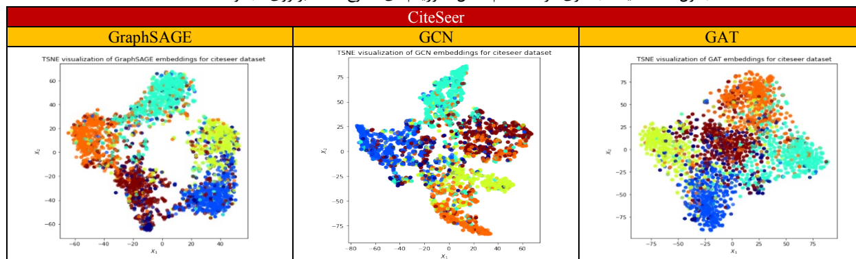
جدول (۵): مقایسه جاسازی گراف هنگام اعمال الگوریتم‌های متنوع GNN بر روی مجموعه داده CiteSeer
