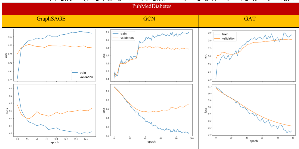
جدول (۲): مقایسه معیارهای Accuracy و loss در زمان‌های Train و Validation بر روی نمودار هنگام اعمال الگوریتم‌های متنوع GNN بر روی مجموعه داده PubMedDiabetes
