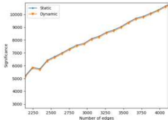
شکل(۶-۶): مقایسه‌ی الگوریتم پویا و ایستای مبتنی بر معیار اهمیت
