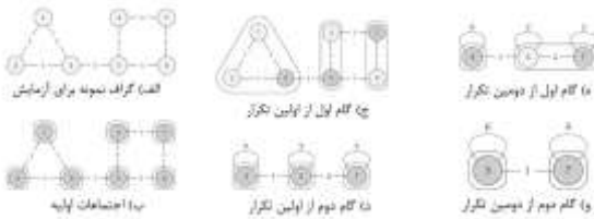
شکل (۶-۲): مراحل روش لووین
