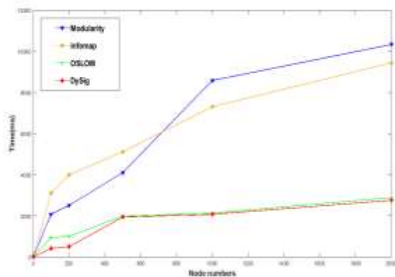
شکل(۶-۷): مقایسه‌ی زمان اجرای الگوریتم‌های مختلف
