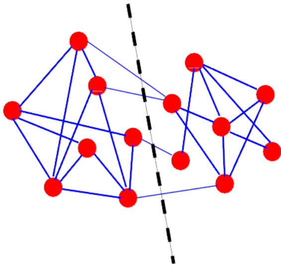
شکل (۵-۱): تقسیم‌بندی گراف به دو گروه هم‌اندازه
