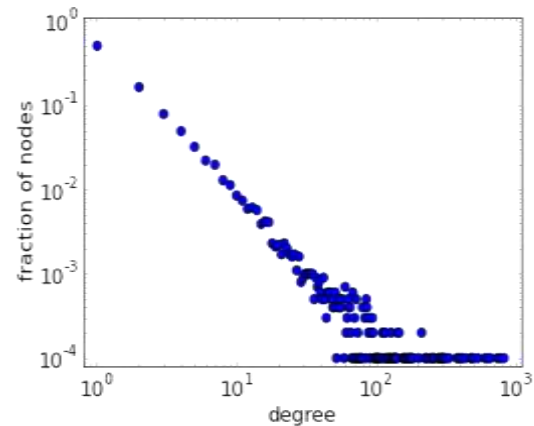
شکل (۳-۱): توزیع درجه‌ی یک گراف با قاعده‌ی توانی [۴]
