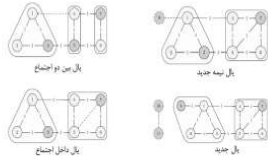
شکل (۳-۶): انواع یال های افزایشی به گراف
