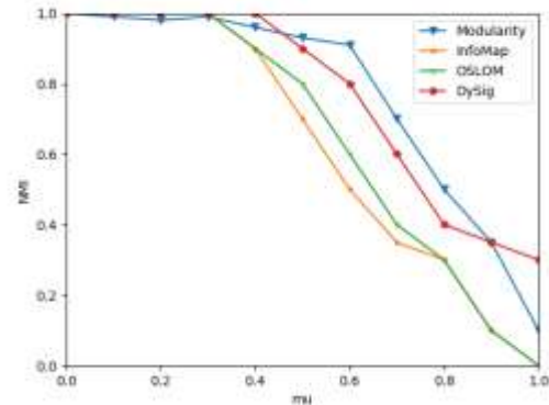
شکل(۶-۵): مقایسه‌ی NMI الگوریتم‌های Infomap, Modularity
