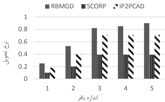
نمودار (۷). نمودار مقایسه نرخ تحویل با تغییر اندازه بافر
