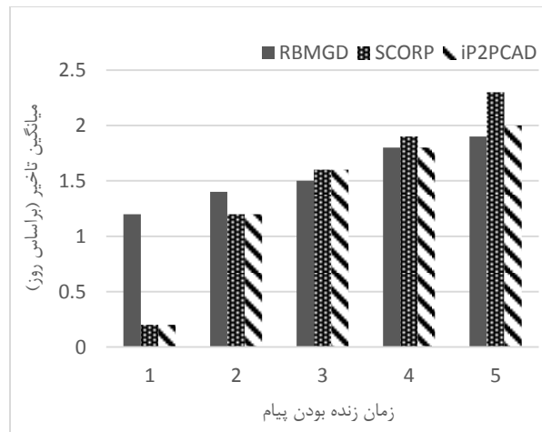
نمودار (۵). نمودار میانگین تأخیر با افزایش زمان زنده‌بودن پیام
