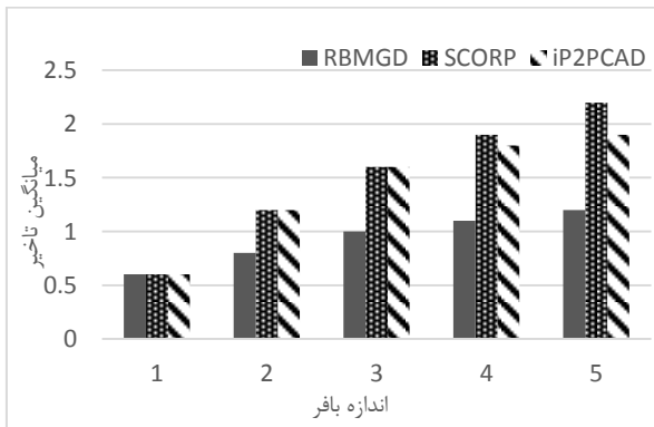
نمودار (۸). نمودار مقایسه میانگین تأخیر تغییر اندازه بافر
