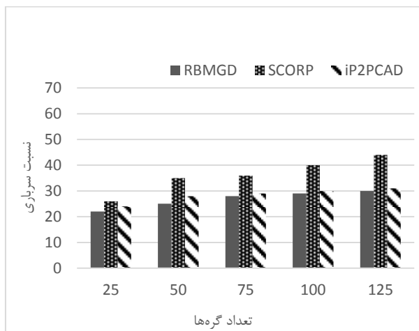
نمودار (۳). نمودار نسبت سرباری با افزایش تعداد گره‌ها
