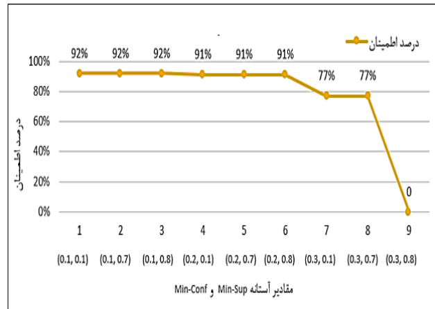
شکل (۹): اطمینان قواعد هم‌آبی تولید شده.
