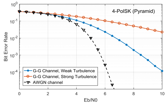
شکل (۷): احتمال خطای بیت بر حسب نسبت انرژی بیت به نویز دریافتی در حالت منظومه ۴ تایی.
